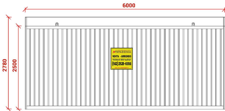
Elevación Norte
