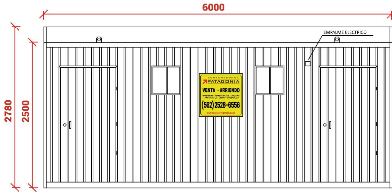
Elevación Sur
