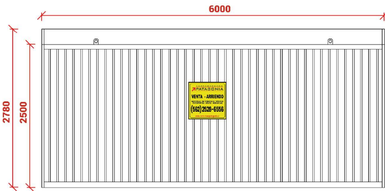
Elevación Norte
