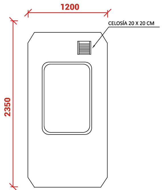
Elevación Sur
