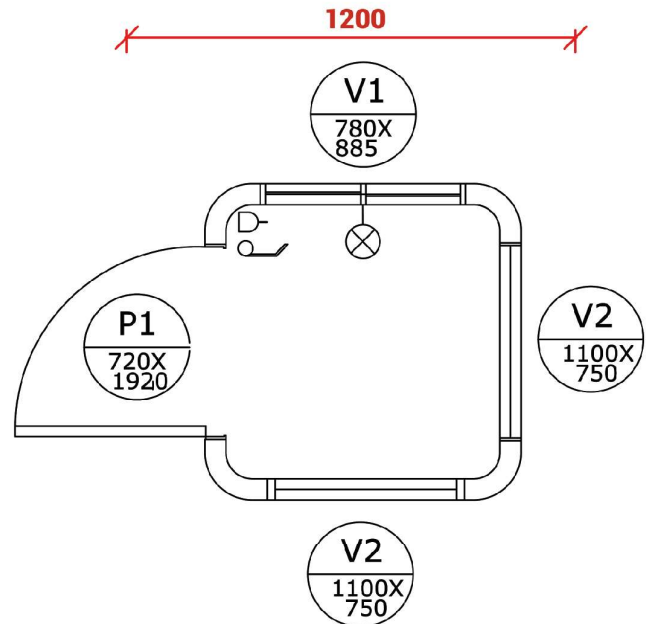
Planta
