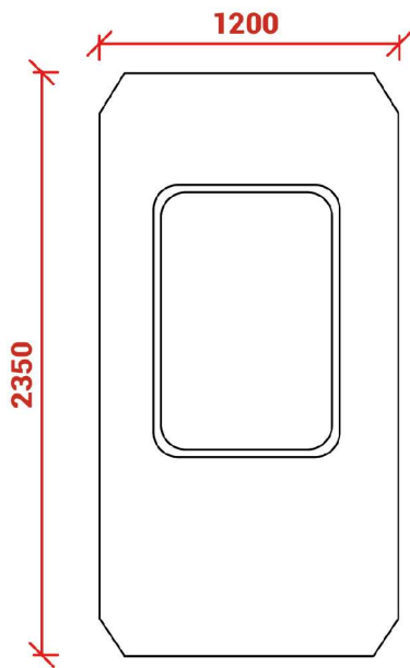
Elevación Este
